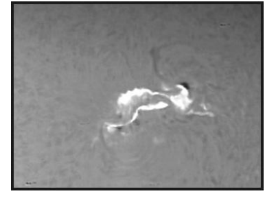
Solar Corona
