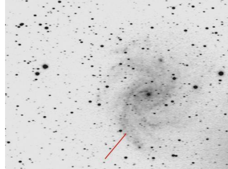
Arp29 - Cepheus NGC6946
